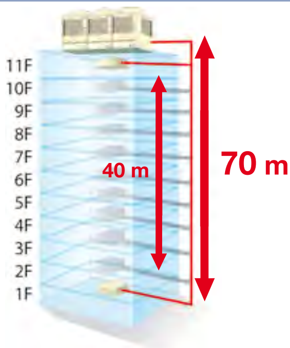
Höhenunterschied zwischen dem Außengerät und dem letzten Innengerät
